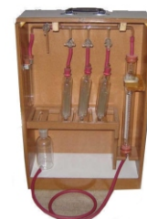
Orset Apparatus
